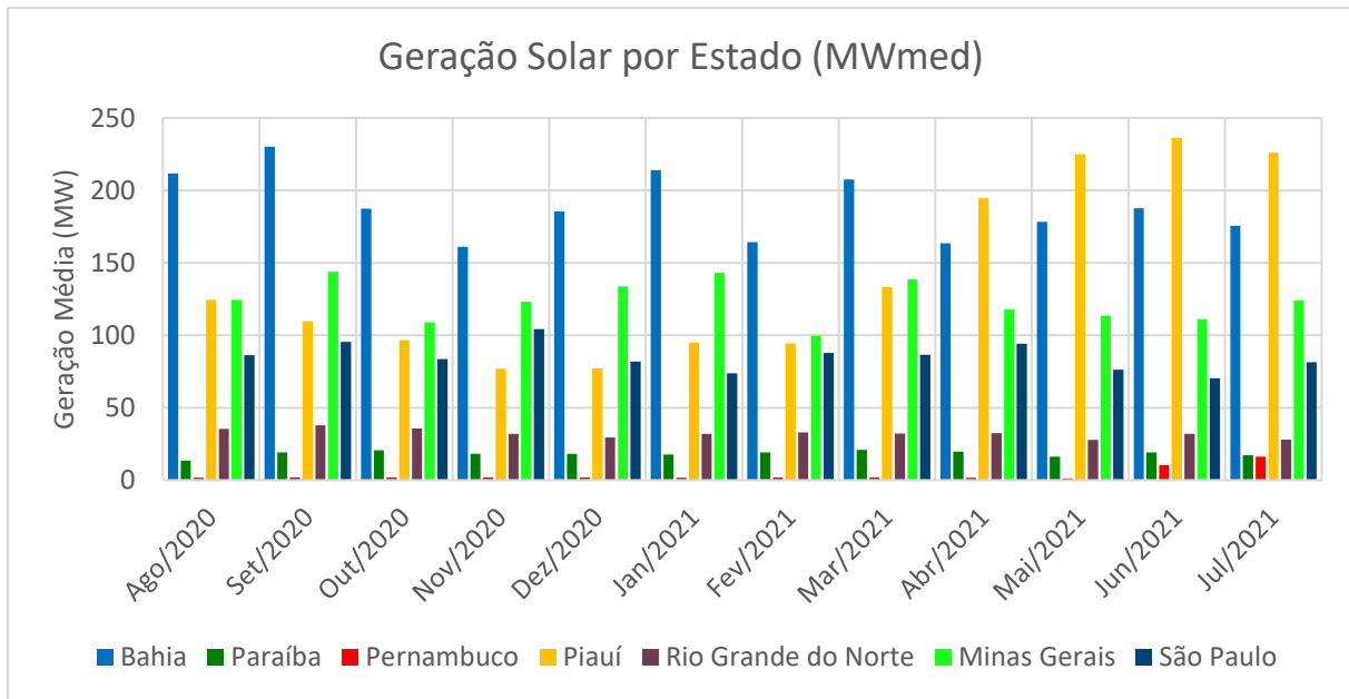
Figura 7 – Geração solar fotovoltaica média mensal (MWmed) nos últimos 12 meses por estado.
